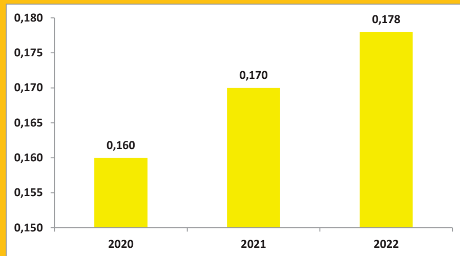
Figura 3.5.1.5 - Indicatore emissioni di CO2 Raffineria di Taranto (kt/kt)
