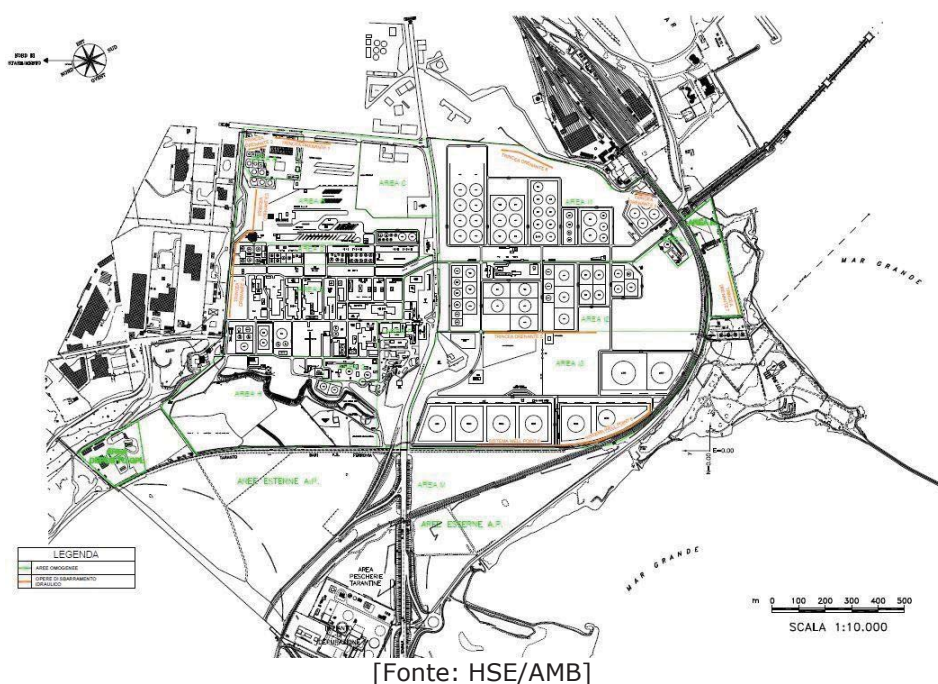
Figura 3.7.3 – Ubicazione Sbarramenti Idraulici di Raffineria
