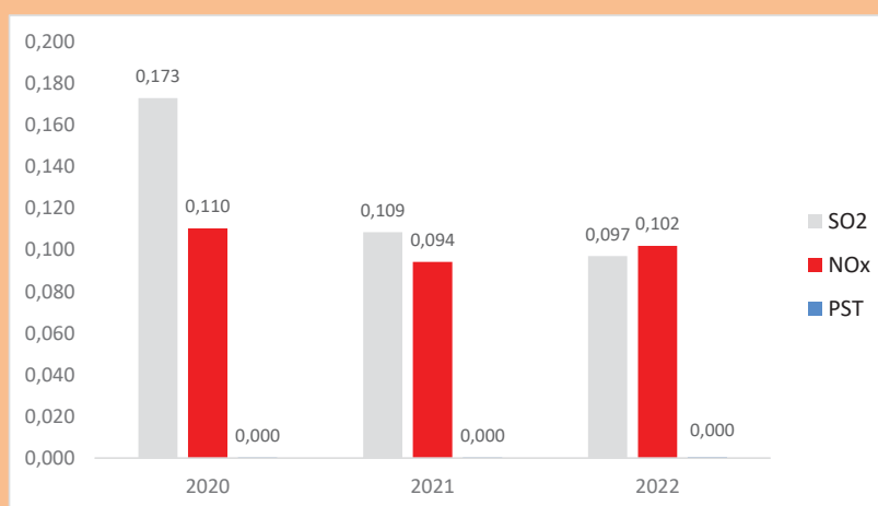
Figura 3.5.1.3 – Indicatore di emissione specifica unitaria Raffineria di Taranto (kg/t)
