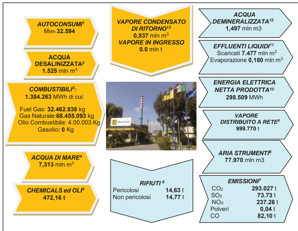
Figura 3.13.1 – Bilancio di massa della Centrale Termoelettrica nel 2022
