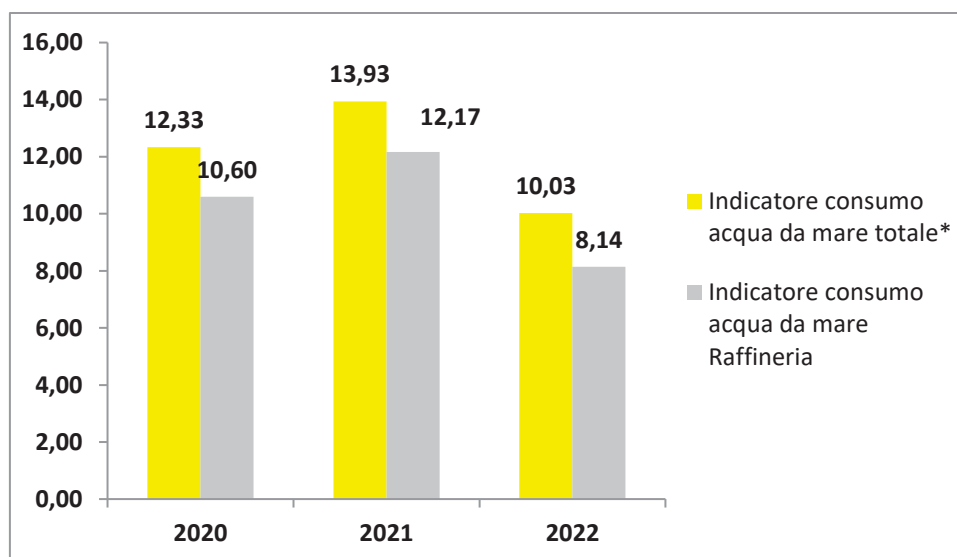
Figura 3.3.1.2 – Indicatore di consumo acqua di mare totale e della Raffineria di Taranto(m 3 /t)
