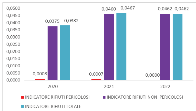
Figura 3.6.2.1 – Indicatori produzione unitaria di rifiuti totale Oleodotto Viggiano - Taranto (t/Kt)
