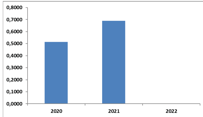
Figura 3.3.2.1 – Indicatore consumo idrico unitario ex Stabilimento GPL di Taranto (m 3 /t)
