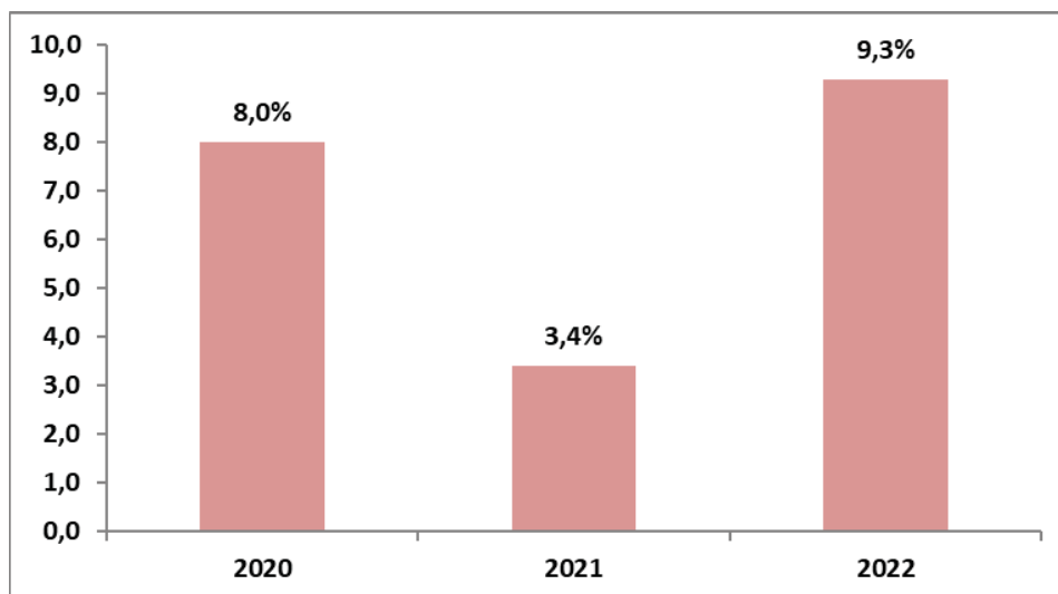
Figura 3.7.2 – Indice situazione piezometri Raffineria di Taranto (%)
