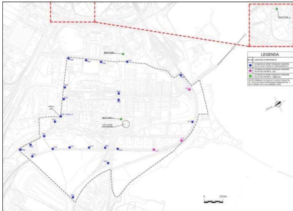
*Figura estrapolata dal Report Impatto Acustico del 31 GENNAIO 2019. [Fonte HSE/AMB]
