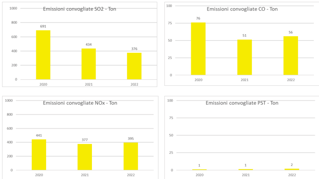
Figura 3.5.1.2 – Emissioni convogliate in atmosfera Raffineria di Taranto (t)
