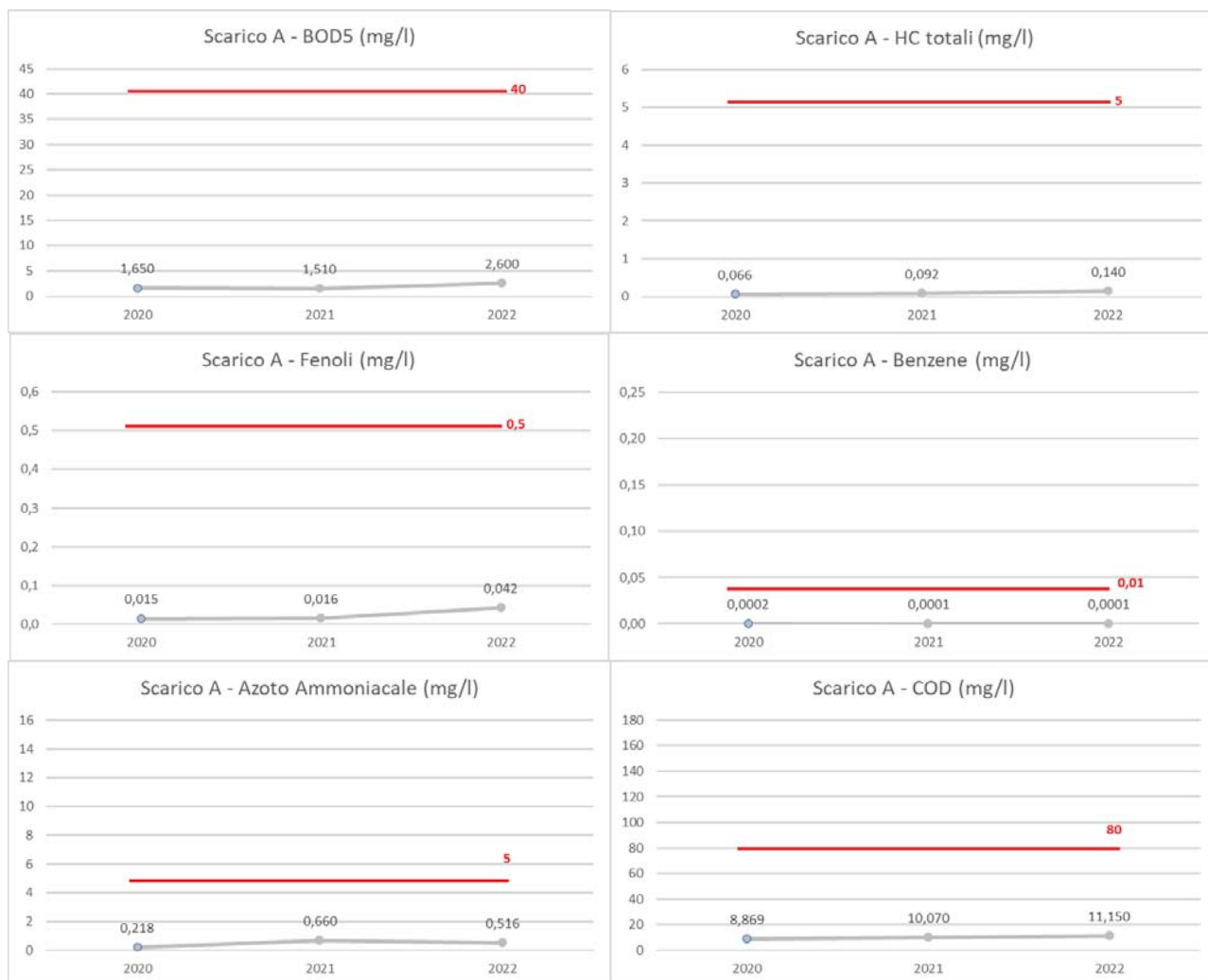
Figura 3.4.1.1 – Qualità degli scarichi idrici nel triennio espressi come concentrazioni medie rispetto ai limiti normativi Raffineria di Taranto (mg/l)
