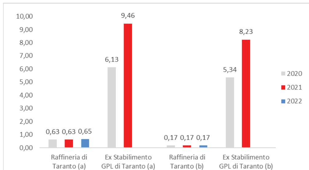
Figura 3.11.1 – Indicatore biodiversità (a,b) Raffineria di Taranto e l'ex Stabilimento GPL Taranto (m 2 /t)
