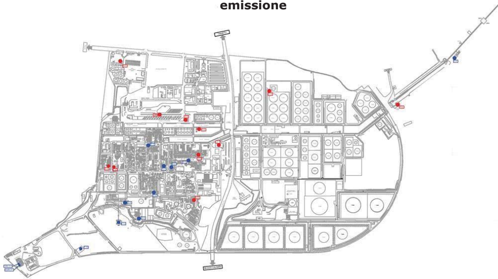
Figura 3.5.1.1 – Planimetria della Raffineria di Taranto con i punti di emissione
